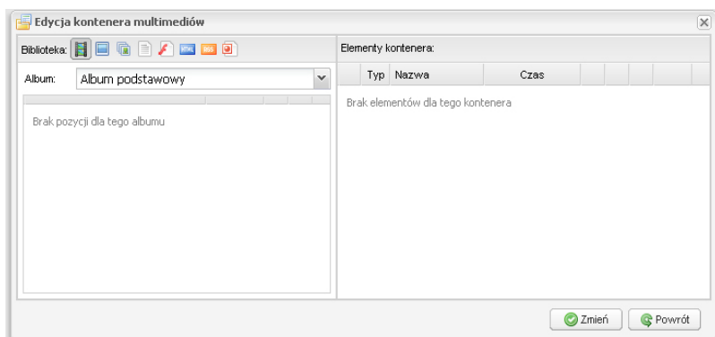
Rys. 47. Widok okna Edycja kontenera multimedii
